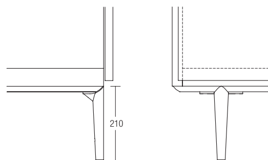
Sezione laterale
