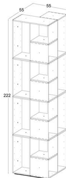
COMPOSIZIONE 9 L55 x h222 x prof.55
