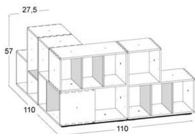
COMPOSIZIONE 4 L110 x h57 x prof.110
