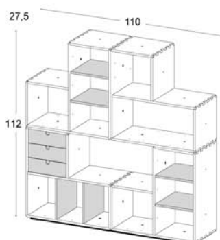
COMPOSIZIONE 11 L110 x h112 x prof.27,5
